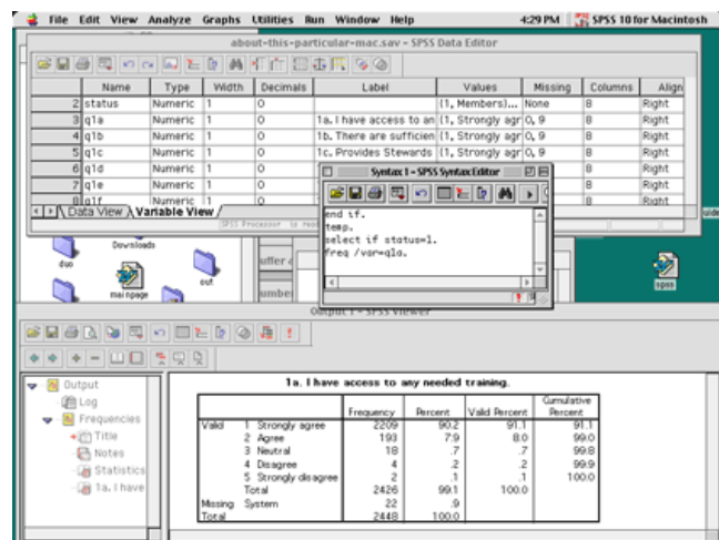
SPSS Workspace
